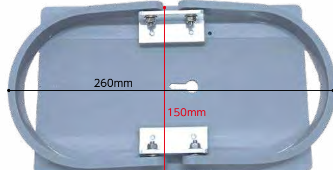
オール塩ビ 改150 踏み台の規格
